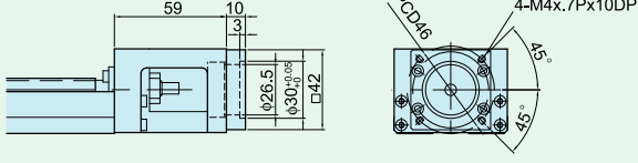
Motor Adaptor Flange F1
