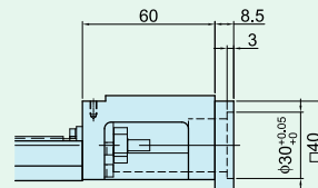
Motor Adaptor Flange F1
